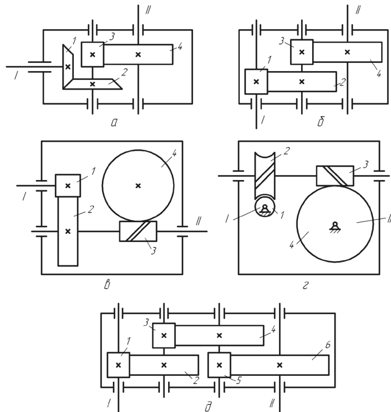
а – коническо-цилиндрический ( i_{\max} = 25 ); б – двухступенчатый цилиндрический ( i_{\max} = 40 ); в – цилиндрично-червячный ( i_{\max} = 150 ); г – двухступенчатый червячный ( i_{\max} = 2000 ); д – трёхступенчатый цилиндрический ( i_{\max} = 200 )
