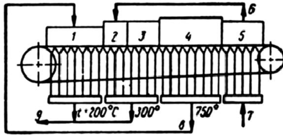
Схема обжига окатышей на конвейерной обжиговой машине
