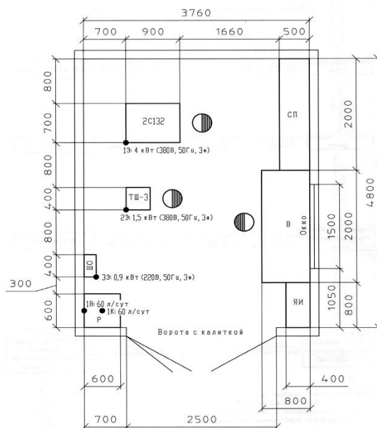
Компоновка мастерской
