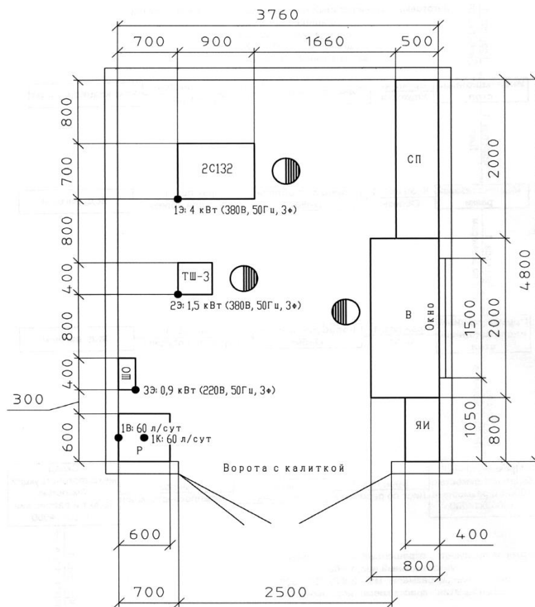
Рисунок 6.3 – Компоновка мастерской
