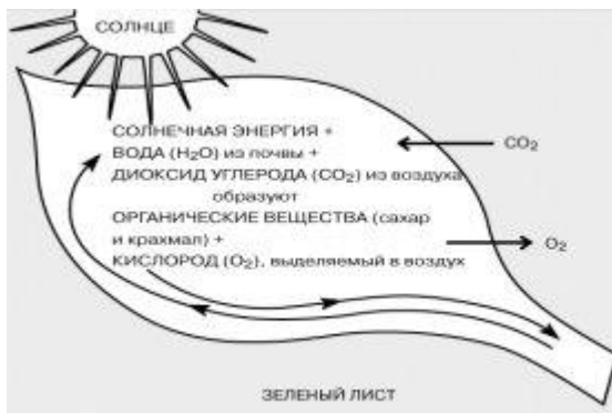
Рисунок 1 – Процесс фотосинтеза
