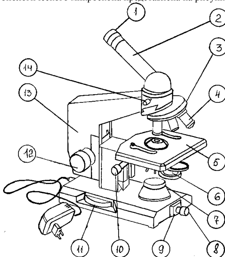
Рисунок 1 – Устройство микроскопа
