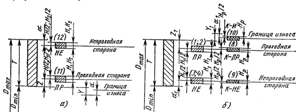
Рис.8. Схемы расположения полей допусков калибров: а - для отверстия; б - для вала
