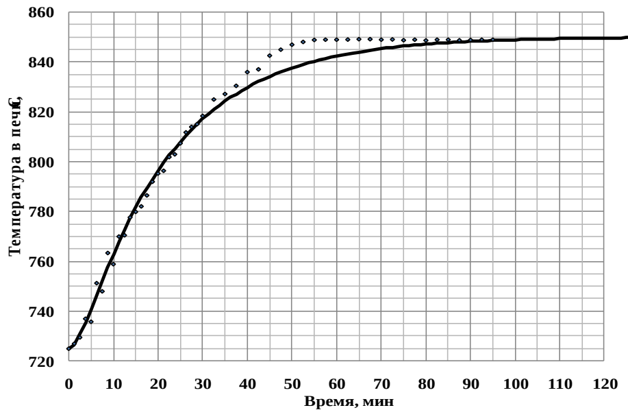
Рис.2 Кривая разгона вращающейся печи
