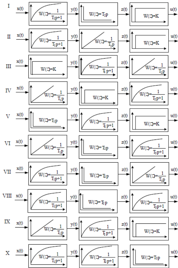
Рис. 2. Структурные схемы по вариантам
