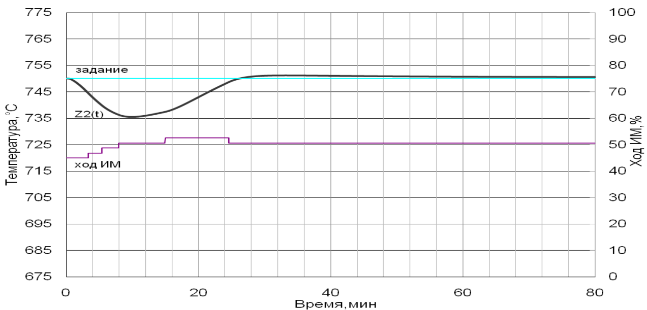
б) регулирование по нагрузке
