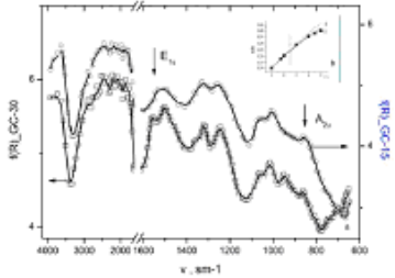
Рис. 1. Спектры диффузного отражения образцов стеклоуглерода (а), концентрационная зависимость интенсивности колебательной моды E_{2g} (б).
