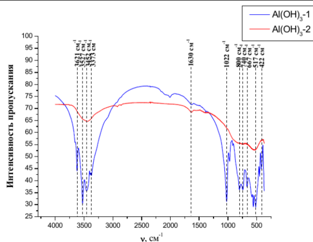
Рис.4.1. ИК спектры гидроксида алюминия Al(OH) 3 -1 и вещества, которое было получено после проведения термogrавиметрического анализа Al(OH) 3 -1 (образ. Al(OH) 3 -2). Спектры сняты с таблеток в КВТ.
