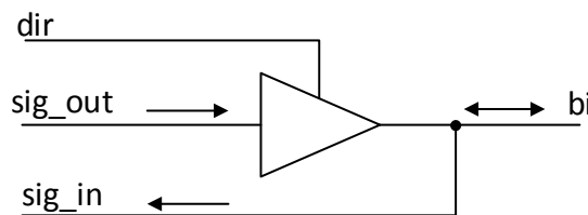
Рисунок 2.2 – Двунаправленный порт
