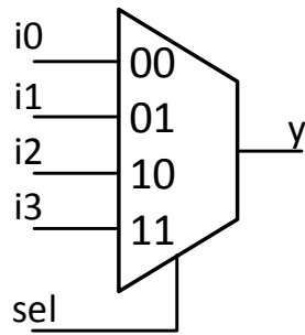
Рисунок 2.6 – Схема мультимплектора 4 в 1
