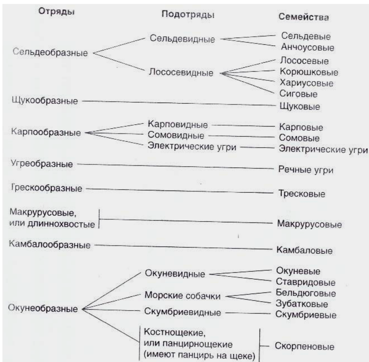
Рис. 2 Фрагмент систематики костистых рыб
