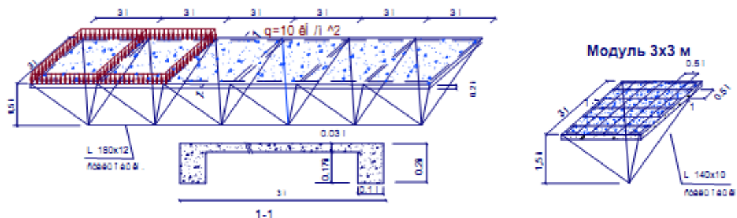
Расчетная схема
