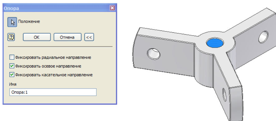
Рис. 6. Задание условий опирания траверсы
