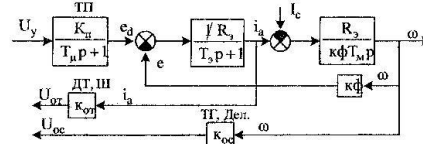
Рисунок 1 – Структурная схема объекта регулирования в СУЭП скорости
