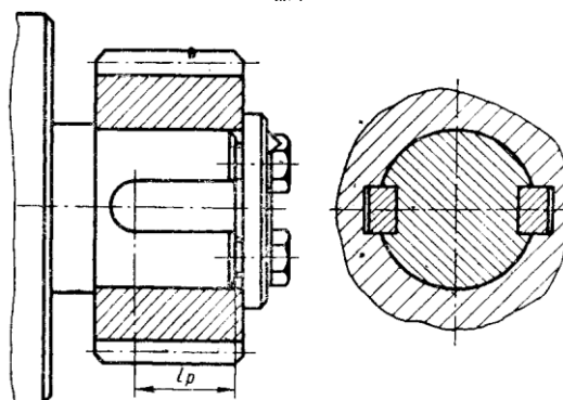
18. Установка шпонок на хвостовой части вала рис. 9
