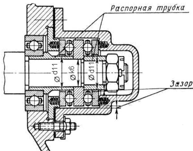
10. Конструирование подшипниковых узлов
