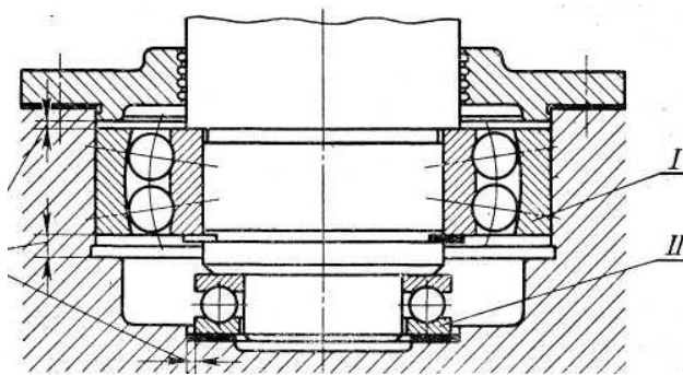
9. Конструирование подшипниковых узлов
