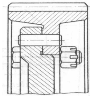
17. Центрирование с использованием штифтов
