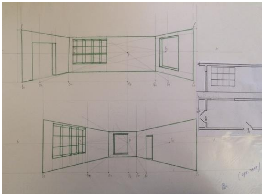
Рис.6. Построение перспективы интерьера методом широкоугольной (широкоформатной перспективы) перспективы
