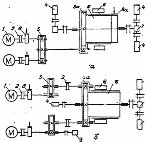
Рис. 3.2. Кинематические схемы скиповых лебедок: а – с общим редуктором; б – с отдельными редукторами
