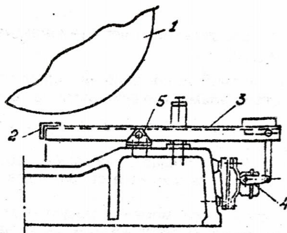
Рис. 3.4. Выключатель слабины каната
