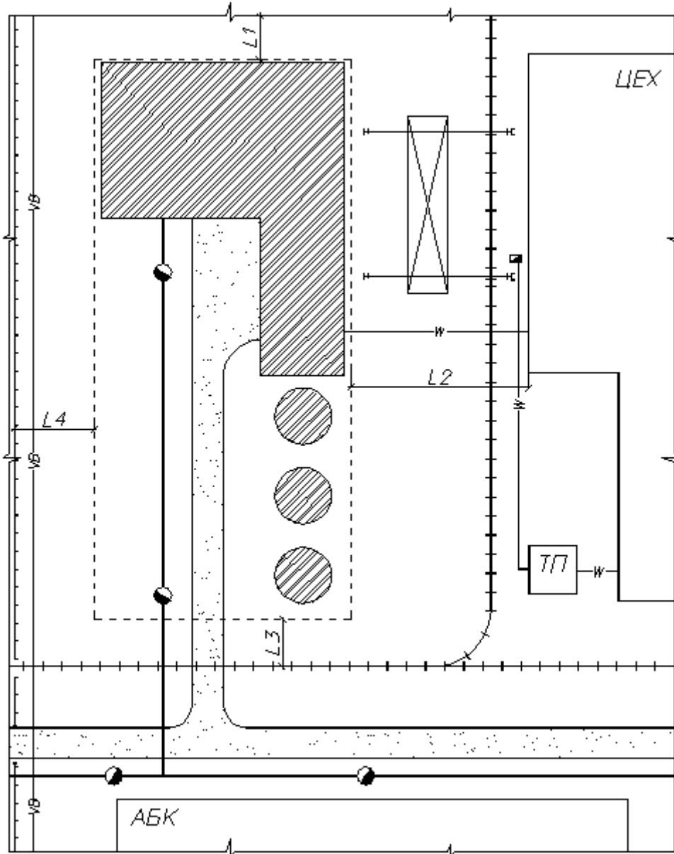
Рис. 5. Схема Генплана одноэтажного промздания (вариант 1)
