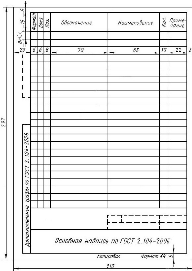
Рис. 3.5. Общая форма спецификации по ГОСТ 2.106-96 ЕСКД
