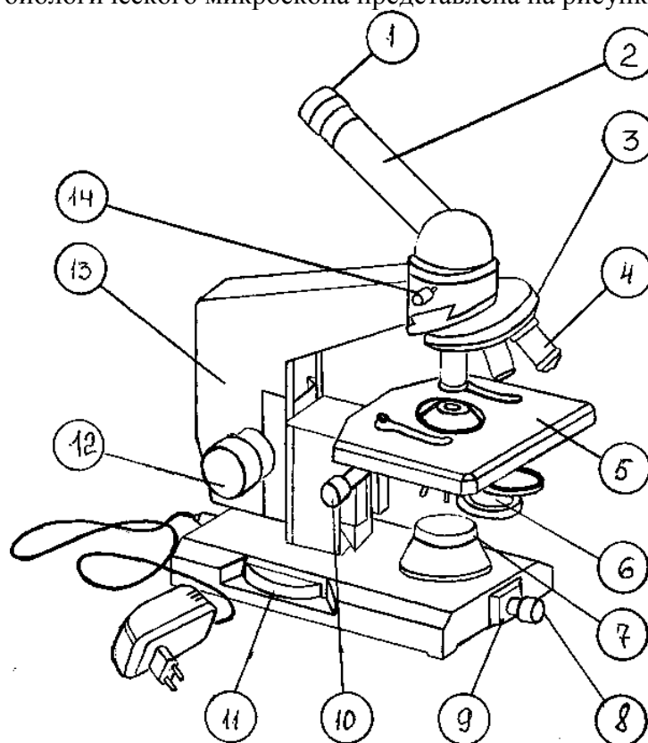
Рисунок 1 – Устройство микроскопа
