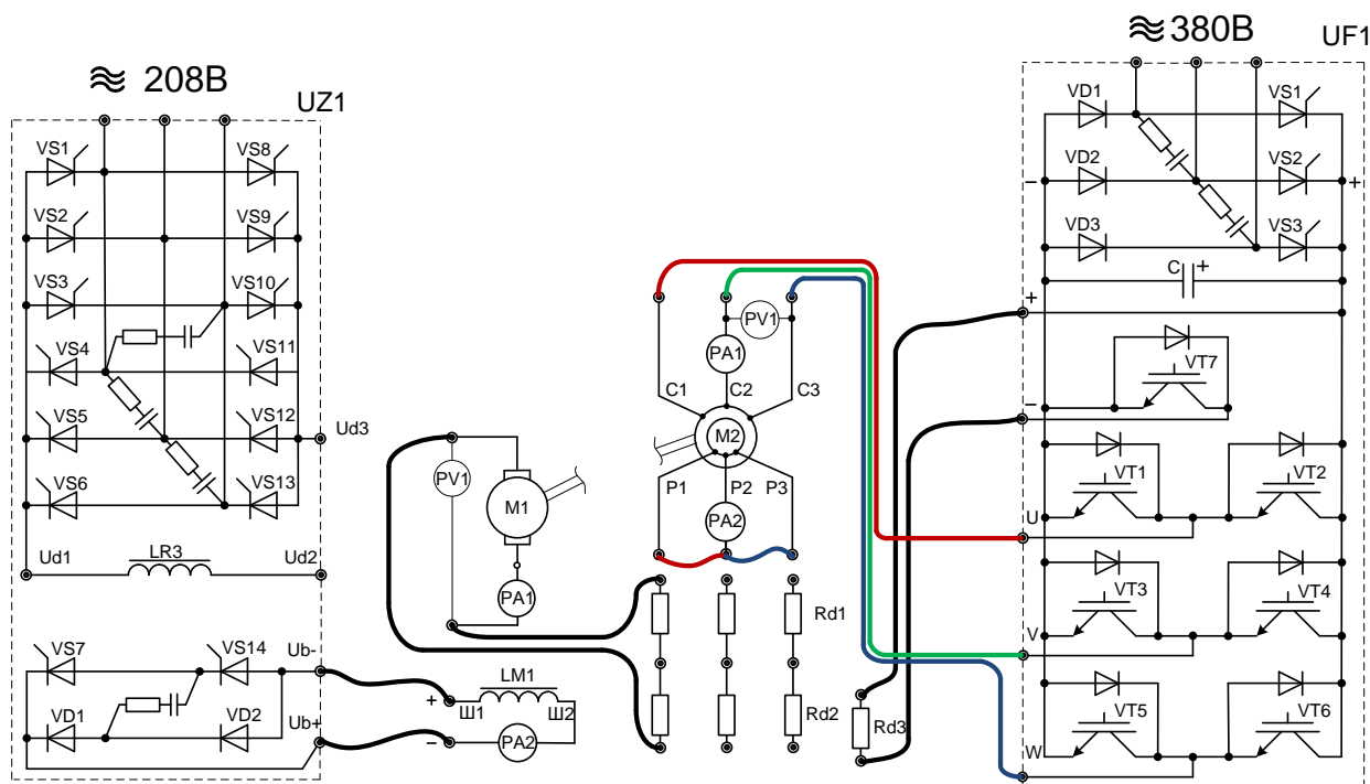
Рис. 1. Силовая схема для снятия переходных процессов i_{\text{я}} = f(t) , n_{\text{об}} = f(t) с добавочным сопротивлением в якорной цепи R_{d\Sigma} = R_{d1} + R_{d2}
