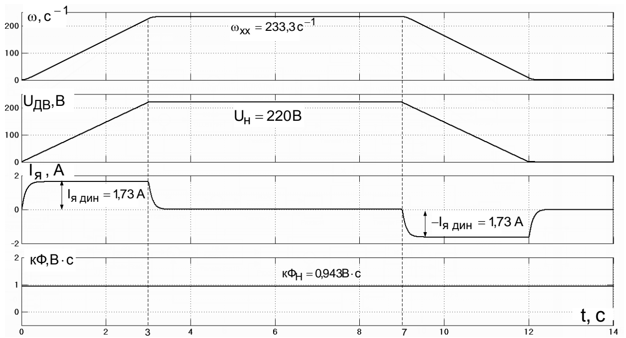
Рис. Переходные процессы привода в режиме x/x в первой зоне регулирования скорости
