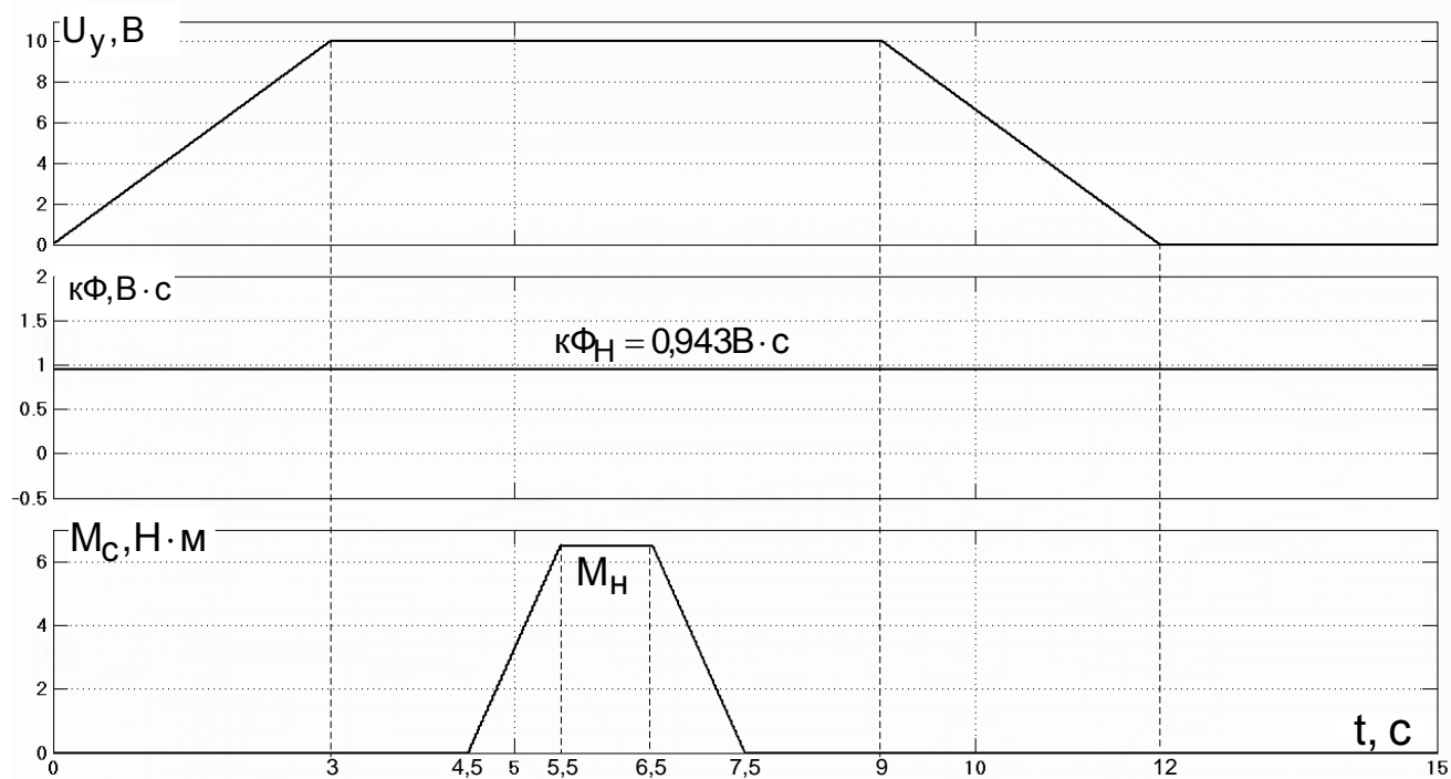
Рис. 2.35. Переходные процессы привода с ударным приложением статического момента во второй зоне
