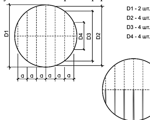
Рисунок 17. Развертка сферы с 6 сегментами
