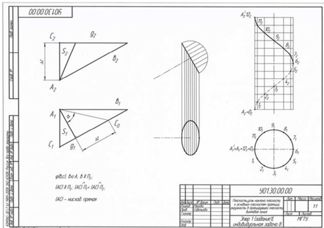
Эпюр №2 «Пересечение прямой с плоскостью. Поверхность»
