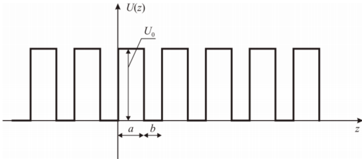
Рисунок 1 – Потенциальный рельеф для электрона в кристалле (модель Кронига–Пенни).
