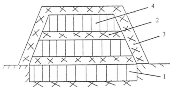
Рис.1. Схема высоконагружаемого полигона ТПО:
