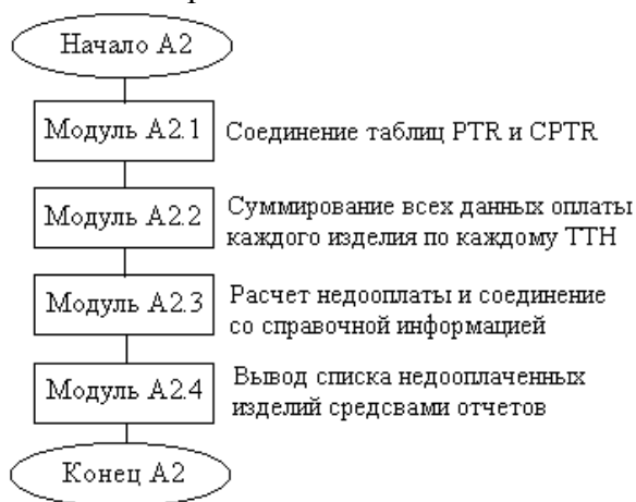
Рис. 5.7. Блок-схема решения подзадачи А2
