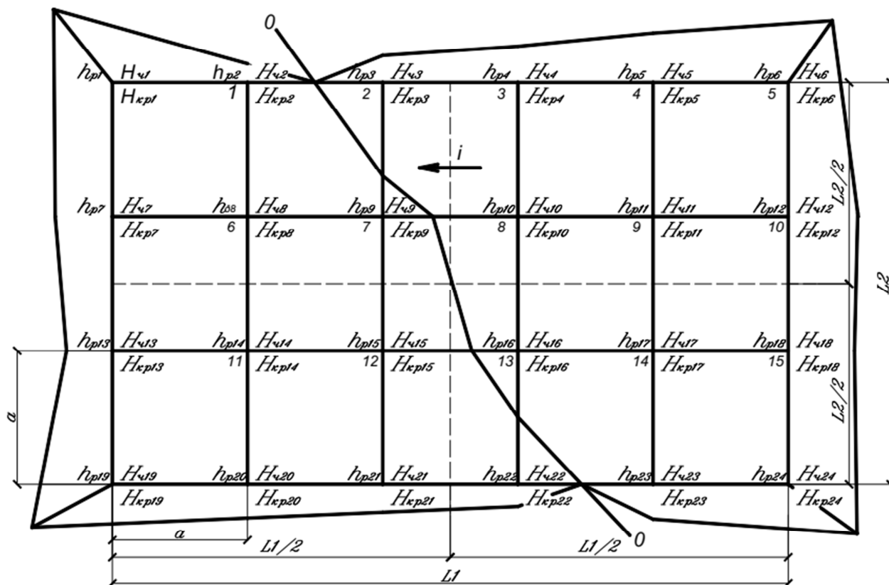
Рисунок 6.2 – План площадки с нанесением черных, красных, рабочих отметок и линии нулевых работ
