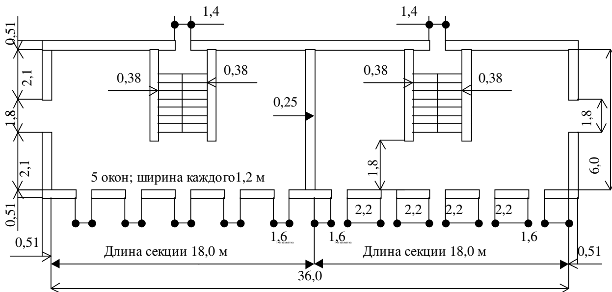
Рисунок 6.4 - План типового этажа
