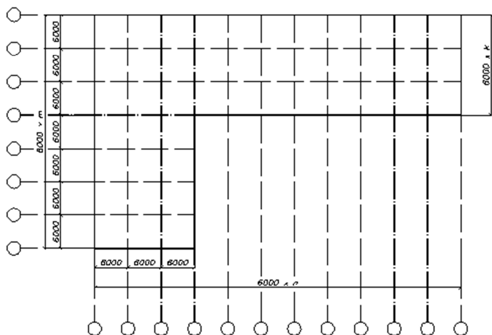
Рис. 1. Схема плана многоэтажного здания
