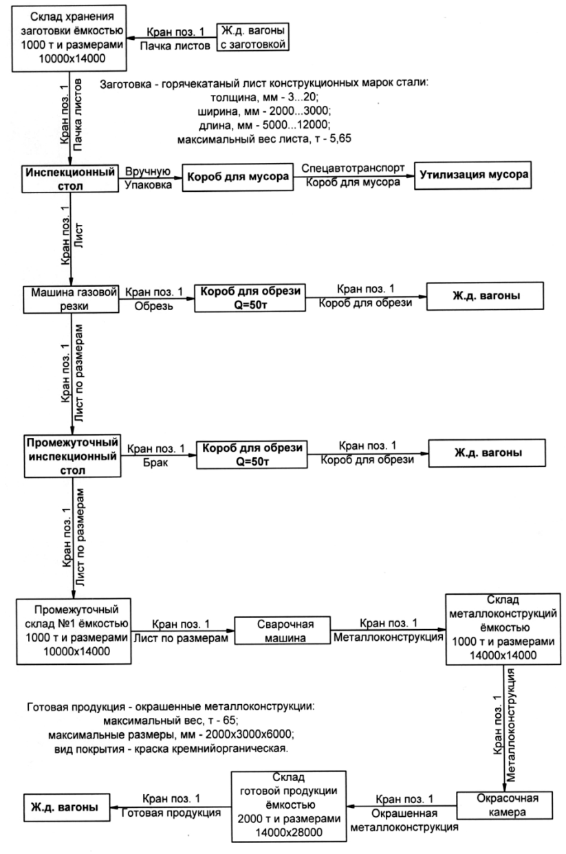
Рисунок 1 - Технологическая схема производства
