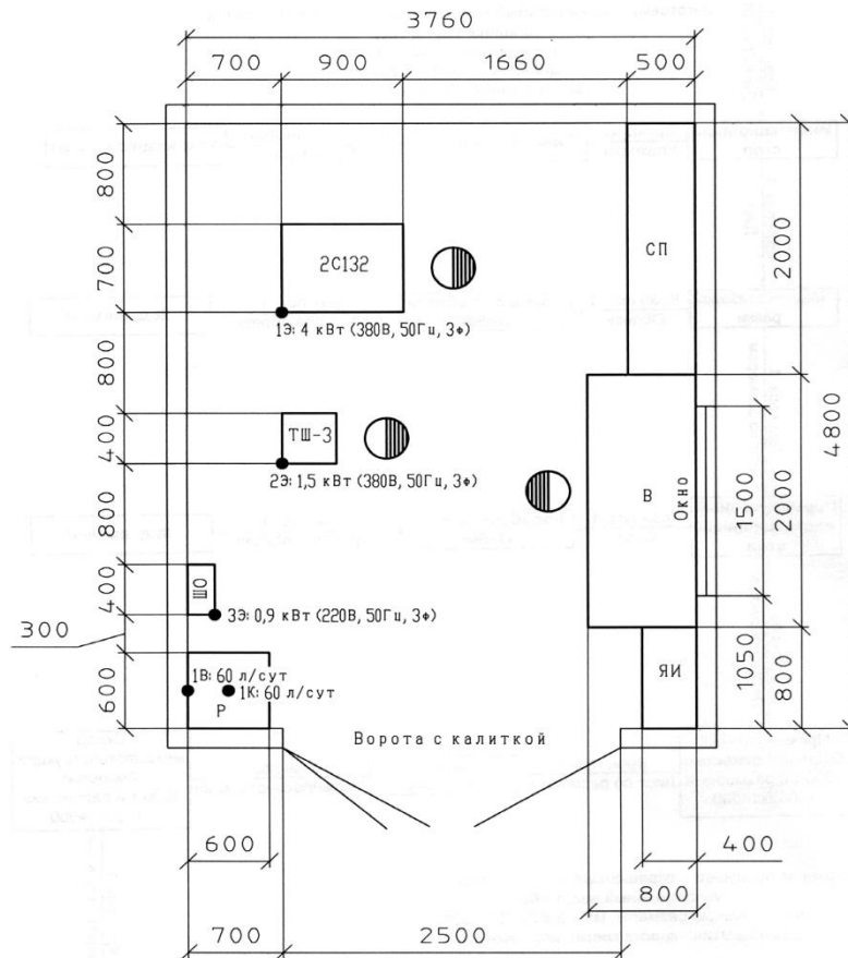
Рисунок 6.3 – Компоновка мастерской
