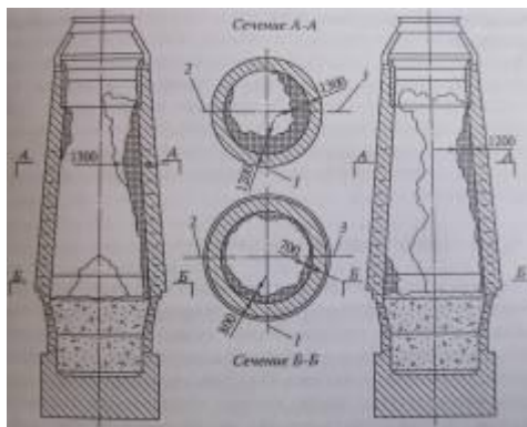
14. Описать представленный способ выкладки лещадки. Дать расшифровку позиций
