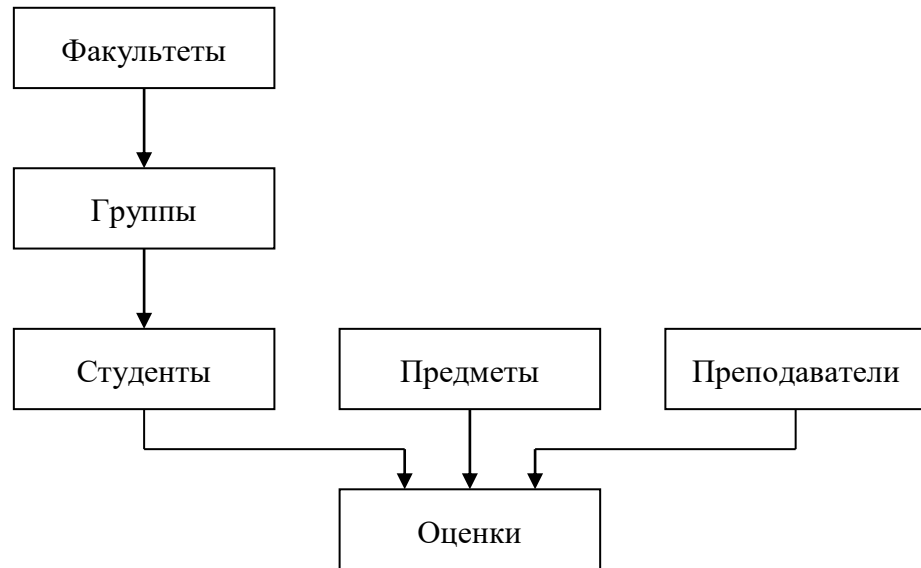
Рисунок 1.1. - Схема структуры предметной области по учету успеваемости студентов
