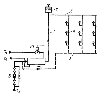
1 — подающий стояк; 2 — воздухоотделитель; 3 — верхний розлив; 4 — разборный стояк; 5 — циркуляционная линия; B — водомер на линии водопроводной воды
