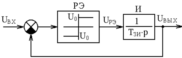
Рис. 2.1. Структурная схема ЗИ
