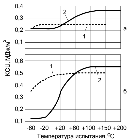
Рис. Вязкость сталей 6XC (1) и 6XB2C (2) в зависимости от температуры испытания: а – закалка на мелкое зерно и отпуск при 250 °С; б – изотермическая закалка при 250 °С
