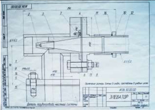
Задание №10 на ПК. «Сборочный чертеж»
