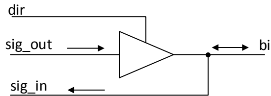
Рисунок 2.2 – Двунаправленный порт
