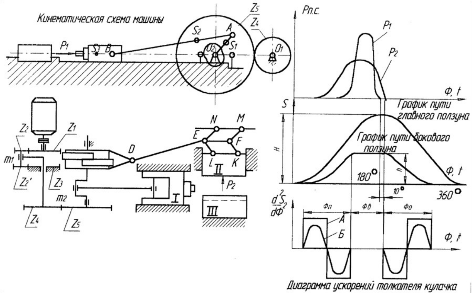
Рис. 3. Горизонтально-ковочная машина
