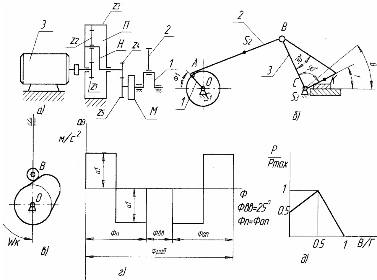
Рис. 2. Механизм ножниц для резки пруткового материала
