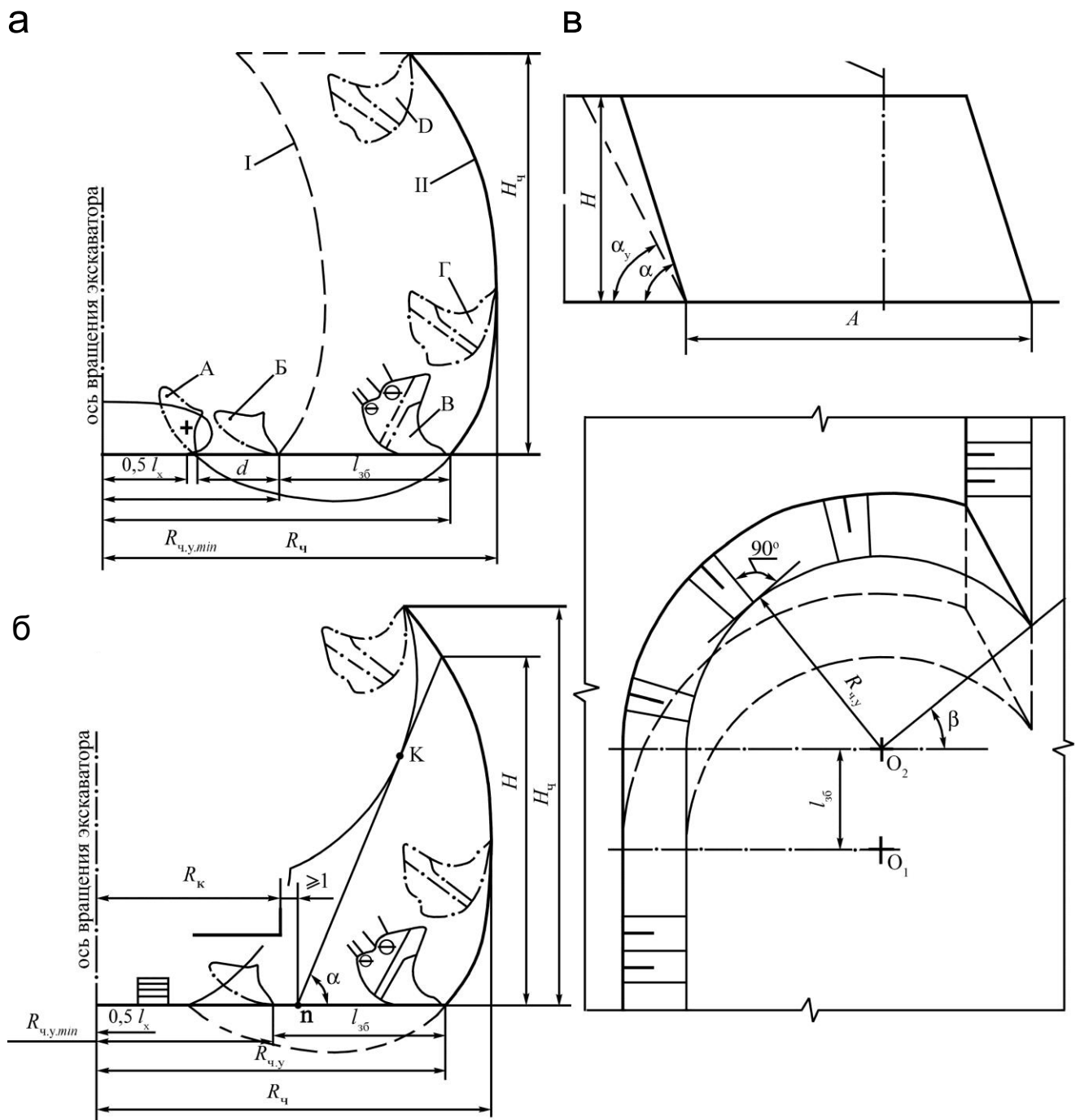
Рис. 3.2 – Отработка забойного блока прямой гидравлической лопаты: а – формирование предельной траектории движения режущей кромки зубьев ковша; б – формирование поверхности откоса уступа сложной заходки; в – изображение откоса забоя в профиле и плане с учетом принятых условностей
