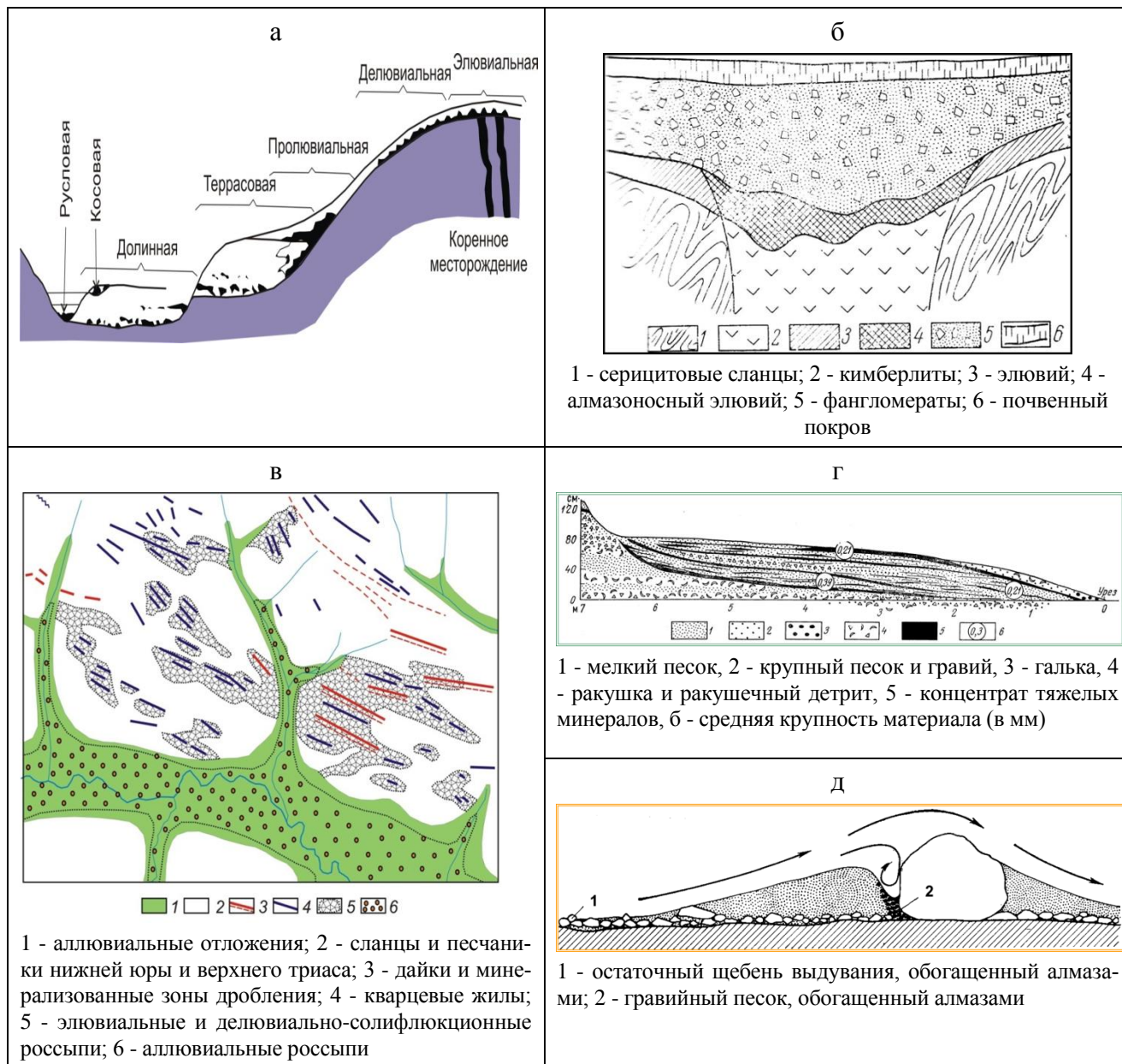
Рис. 1.1 – Условия образования россыпей:
