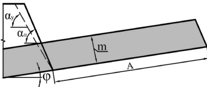
Рис. 3.1 – Параметры заходки по угольному пласту: m – мощность пласта, м; A – ширина заходки, м; α y , α – соответственно устойчивый и рабочий углы откоса уступа, град; φ – угол залегания пласта, град
