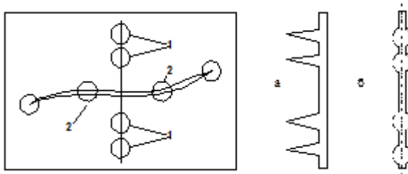
Рис. 2 – Сшивание трещин
