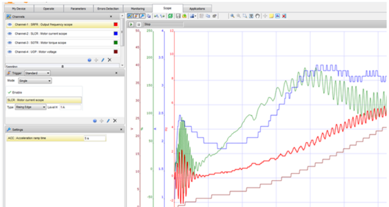
Рисунок 15 – Осциллограммы пуска двигателя
