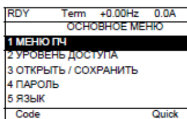
Рисунок 4. Графический терминал. Первое включение ПЧ
