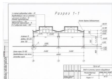
Выполнение работы "Разрез промышленного здания"
