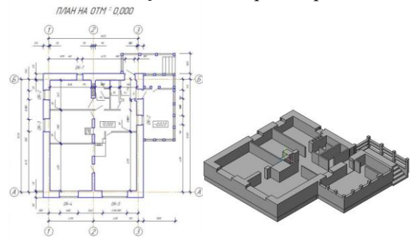
Выполнение работы «Чертеж жилого здания»
