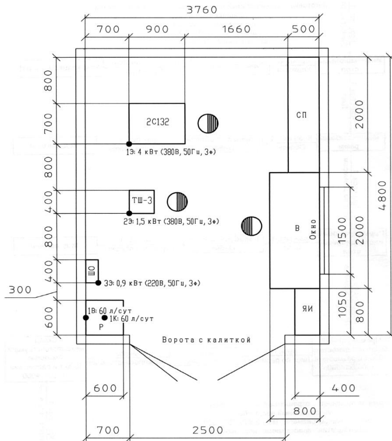
Рисунок 6.3 – Компоновка мастерской
