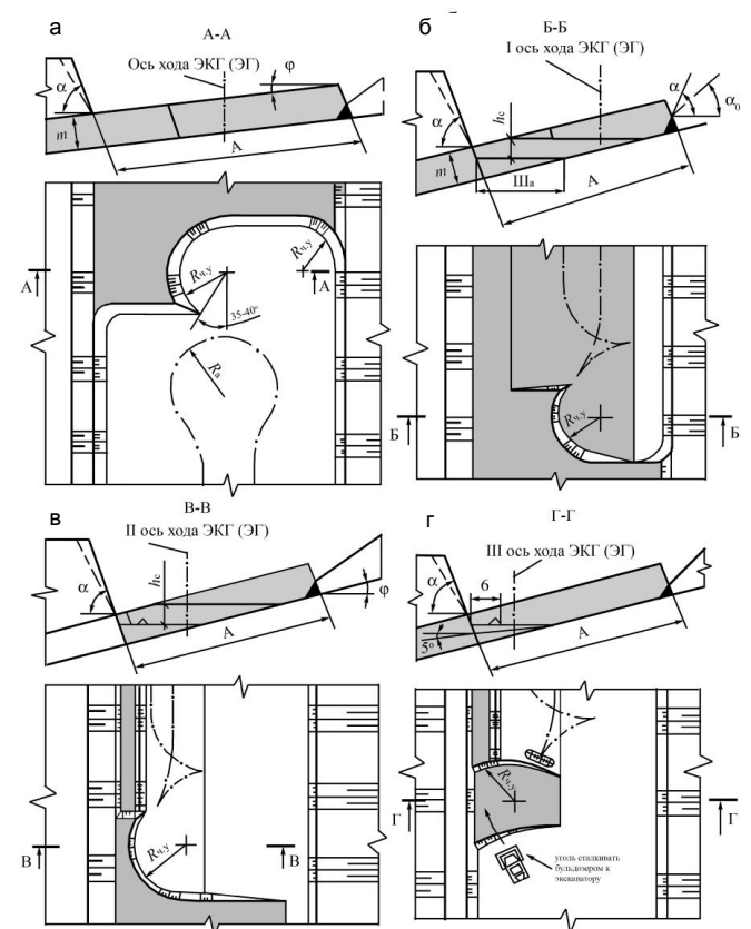
Рис. 3.2 – Варианты разработки мощного пологого пласта:
