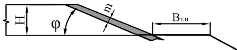
Рис. 6.1 – Параметры залегания наклонного пласта: H – высота вскрышного уступа, м; \phi – угол залегания пласта, град; m – мощность пласта, м; B_{т.п} – ширина транспортной площадки, м
