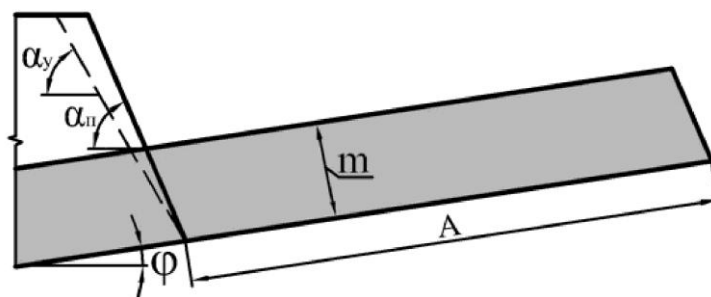
Рис. 3.1 – Параметры заходки по угольному пласту: m – мощность пласта, м; А – ширина заходки, м; α у ,
