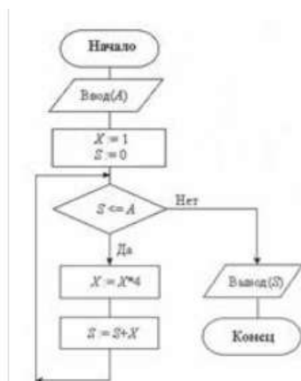
Рис.1. Блок-схема алгоритма
