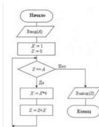
Рис. 1. Блок-схема алгоритма
