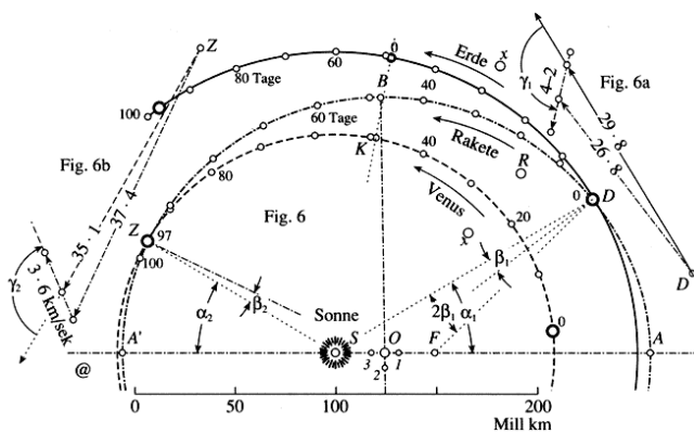
Рисунок 9. График из статьи Гвидо фон Пирке с расчетами траекторий полетов к Венере, 1933 г.
