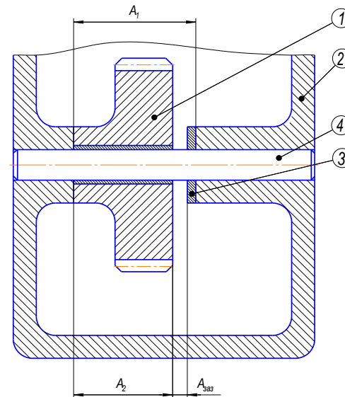
Рисунок - Сборочная единица промежуточного вала редуктора
