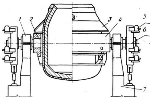
Кислородный конвертер:
