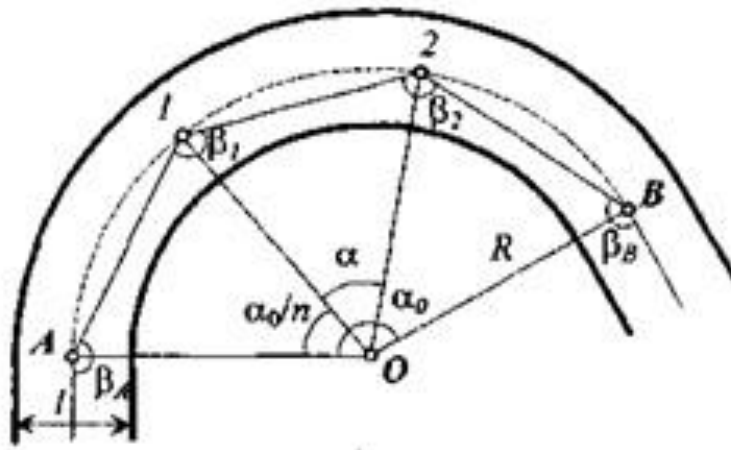
Рис.5.3. Схема закругления
