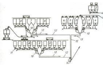
Рис. 5.69. Схема шихтоподачи в доменной печи "Алтай" объемом 2032 м 3 . 1 – бункер окатышей; 2, 3 – бункера известняка; 4 – бункера агломерата и руды; 5 – бункера окатышей и руды; 6, 7 – бункера кокса; 8 – бункера доменного склада; 10 – весовые воронки; 11–13 – питательные весы; 14 – скан.
