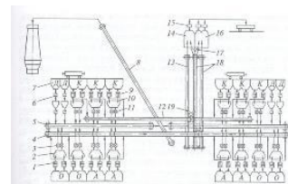
Рис. 5.70. Схема конвейерной шихтоподачи в доменной печи с диаметром шахты 2000 мм.
